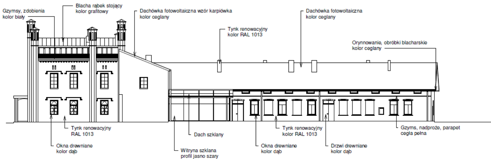
1 Południowo zachodnia 1 : 200
